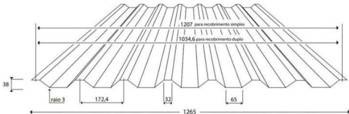
FIGURA 1: MEDIDAS DAS TELHAS TRAPEZOIDAIS PADRÃO ALCOA
