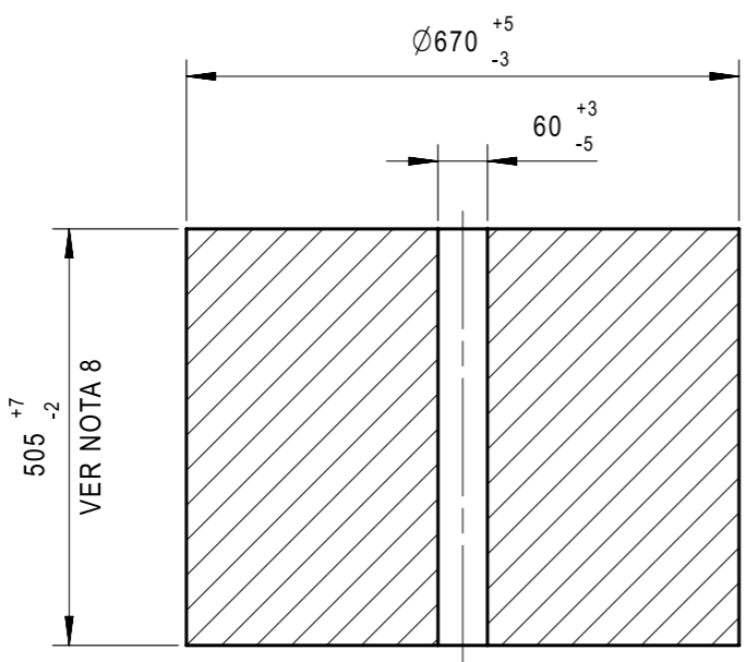
CORTE A-A ESC.: 1:10
