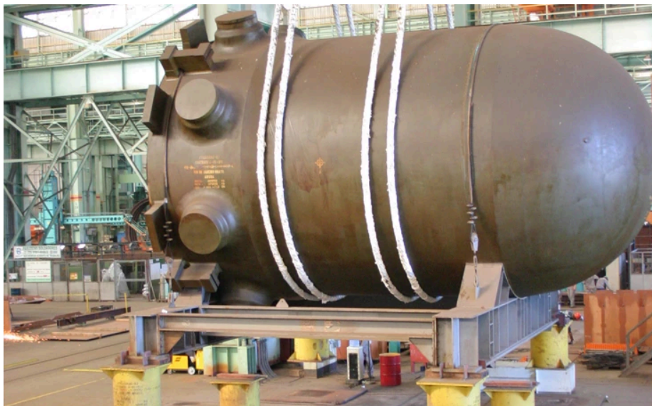
O vaso do reator nuclear do LABGENE. Foto: Nuclep
